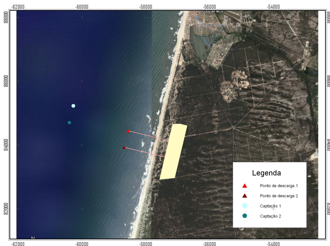
Figura 1.2 – Implantação das tomadas de água e da rejeição de águas residuais.
